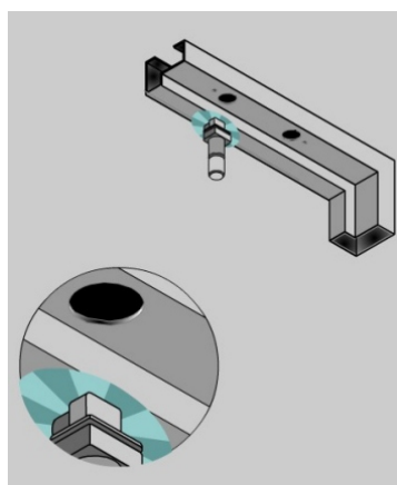
5. 切割鎖體與門門板螺絲位置。
