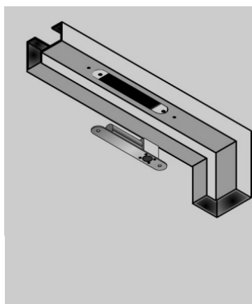
7. 把電插鎖固定在門框上,接上電源,并且測試。
