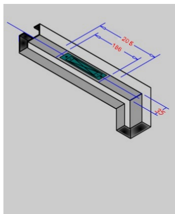
2. 將開孔紙與中心點對齊并且貼上。
